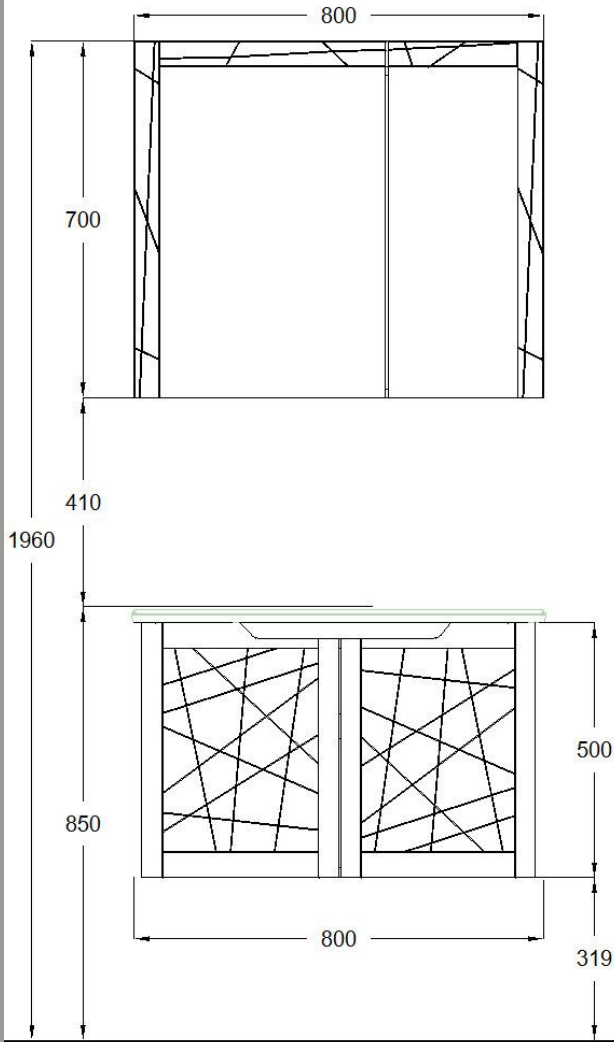
ÖN GÖRÜNÜŞ
