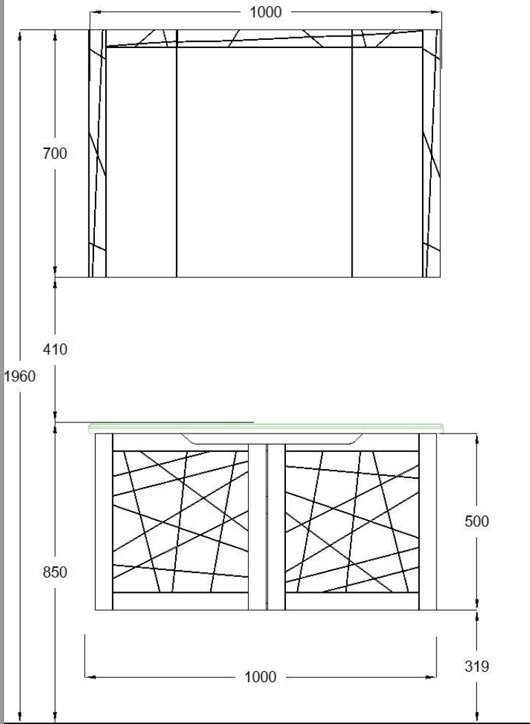
ÖN GÖRÜNÜŞ
