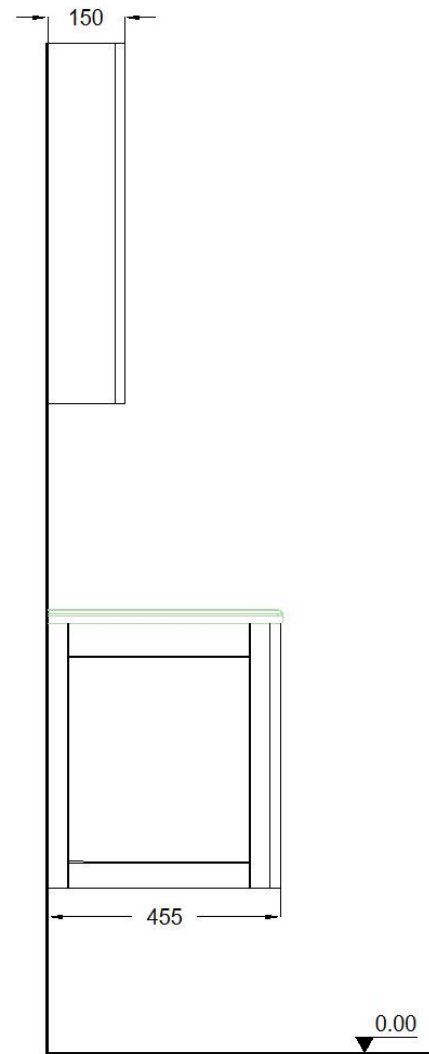
YAN GÖRÜNÜŞ
