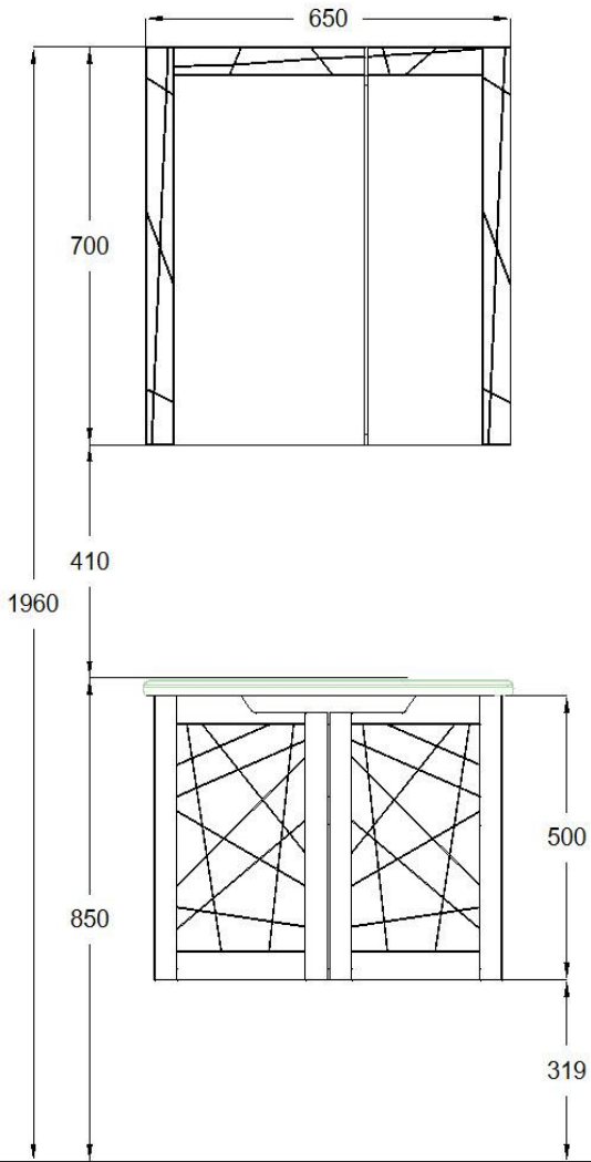
ÖN GÖRÜNÜŞ
