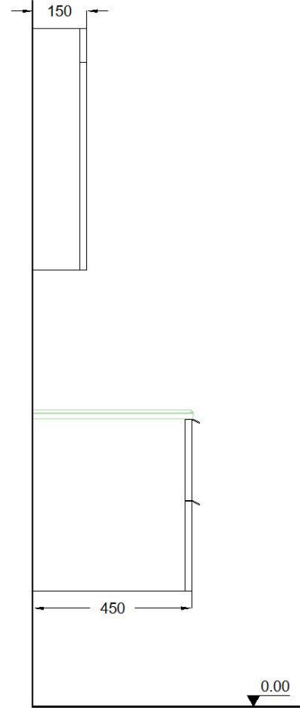
YAN GÖRÜNÜŞ
