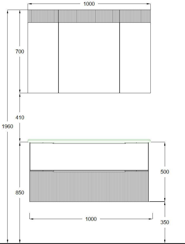
ÖN GÖRÜNÜŞ
